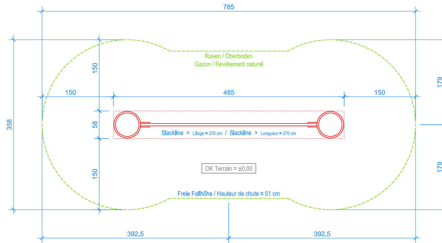
GRUNDRISS / PLAN 1:50
