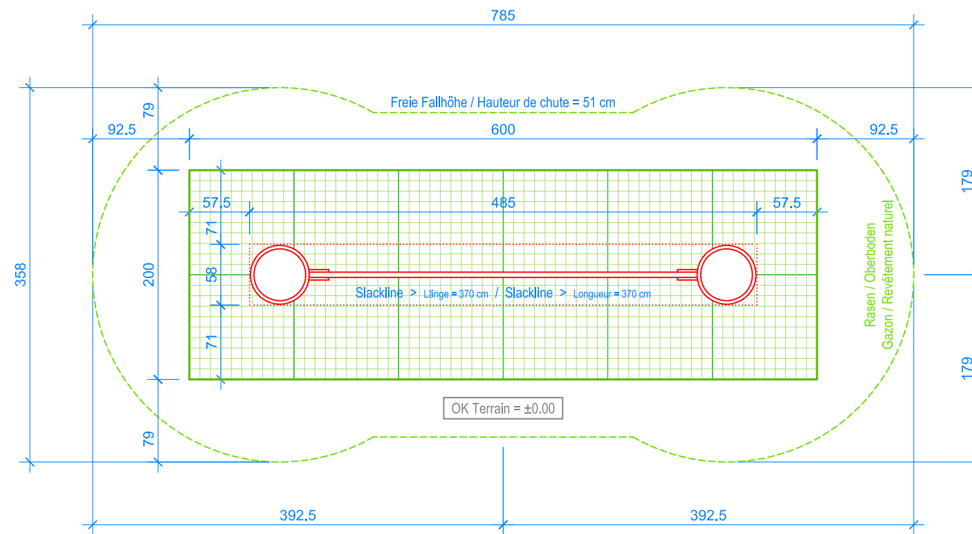
GRUNDRISS / PLAN 1:50
