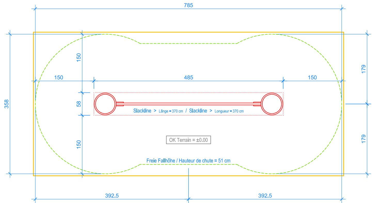
GRUNDRISS / PLAN 1:50
