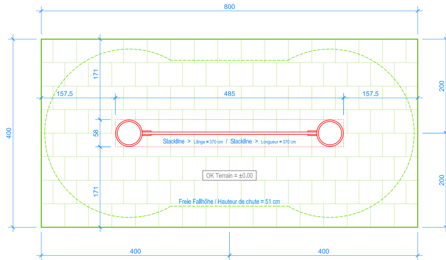
GRUNDRISS / PLAN 1:50
