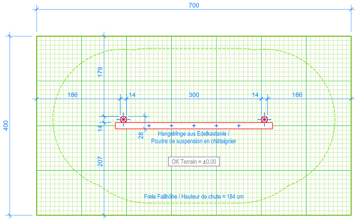
GRUNDRISS / PLAN 1:50
