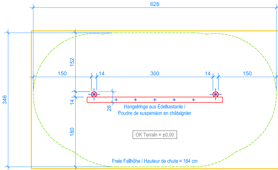
GRUNDRISS / PLAN 1:50
