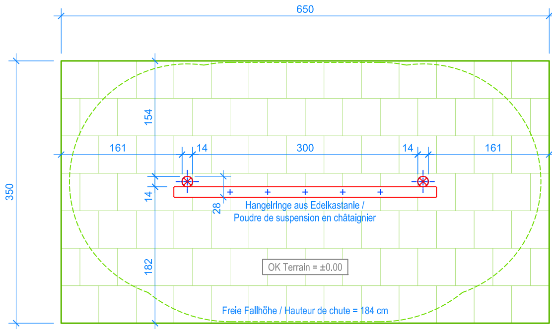
GRUNDRISS / PLAN 1:50
