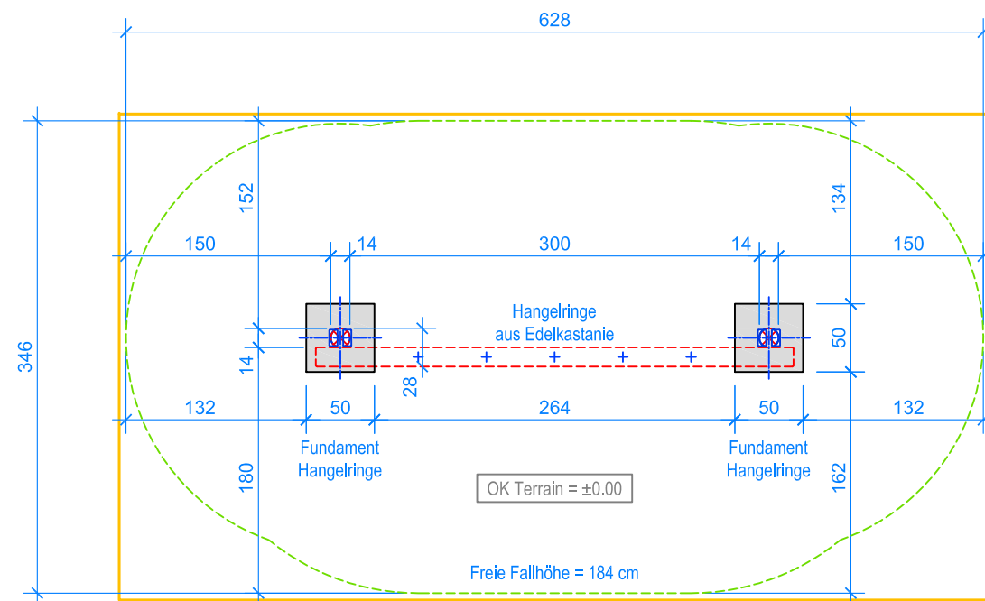
GRUNDRISS 1:50
