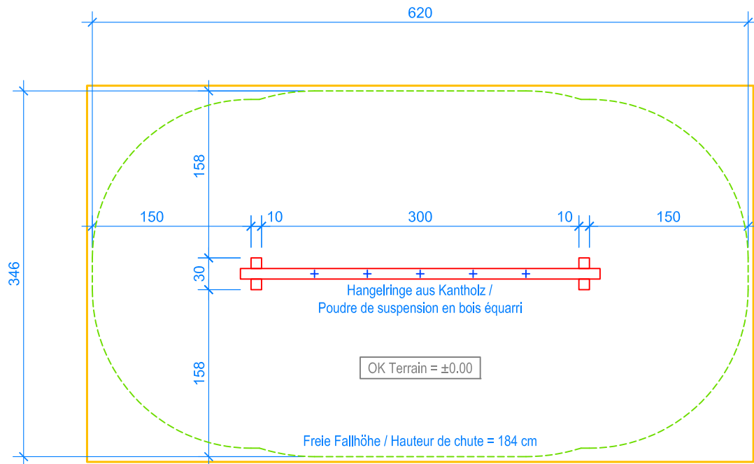
GRUNDRISS / PLAN 1:50
