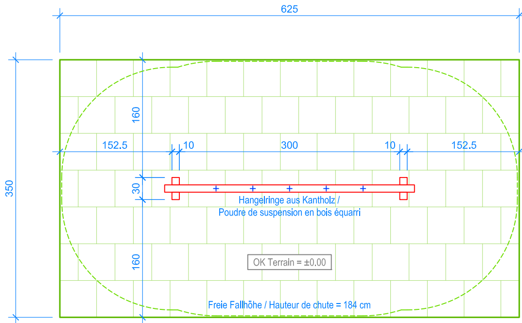
GRUNDRISS / PLAN 1:50
