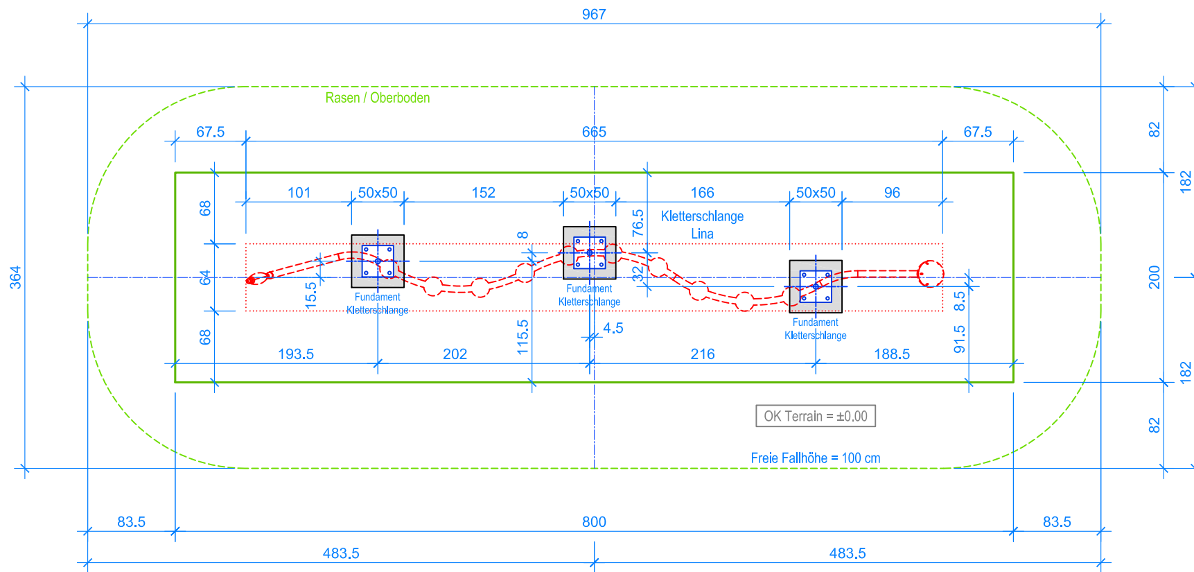
GRUNDRISS 1:50
