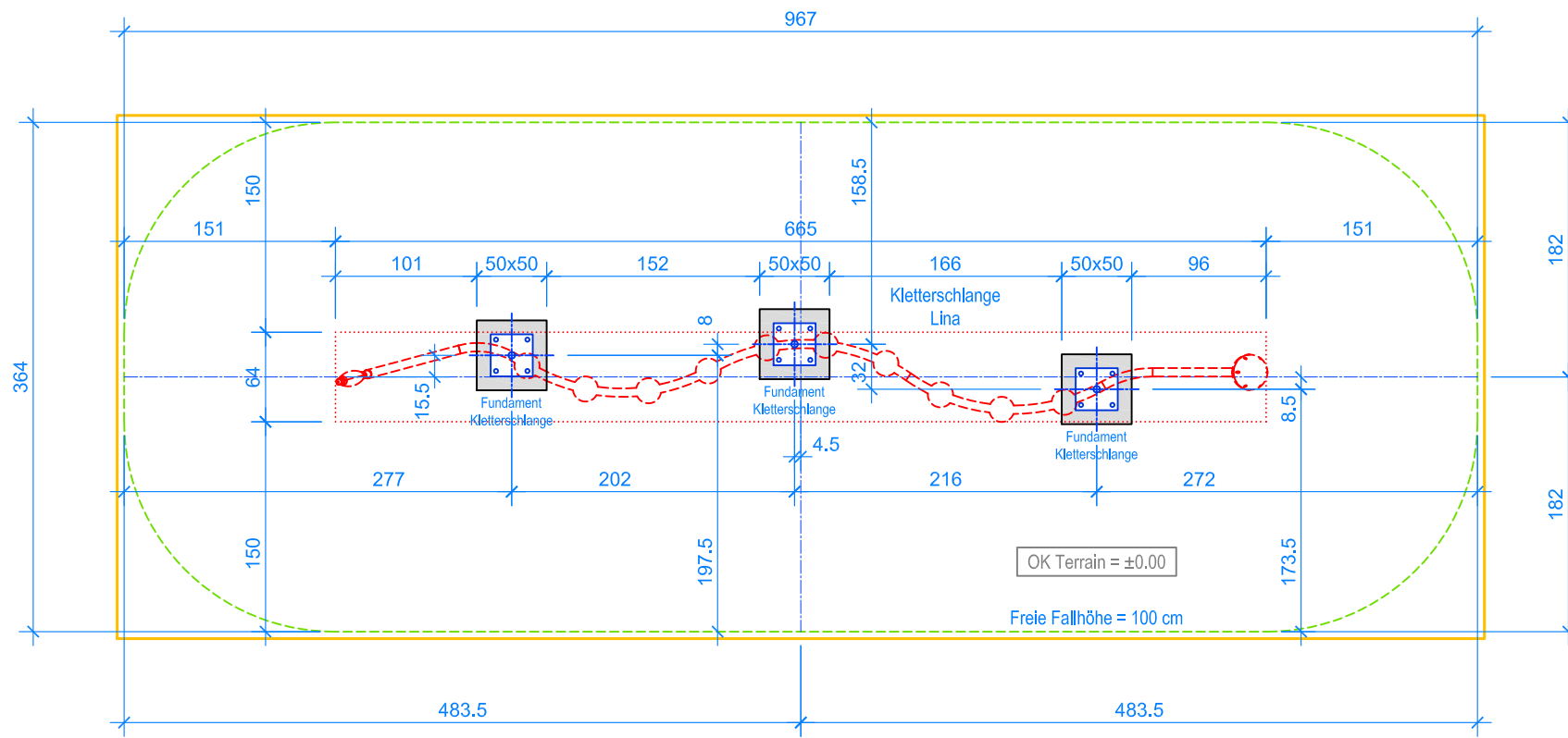
GRUNDRISS 1:50
