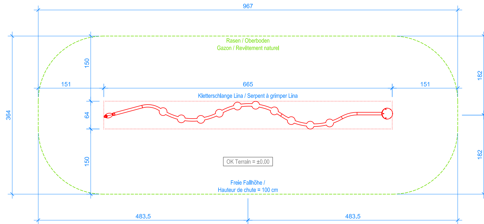
GRUNDRISS / PLAN 1:50
