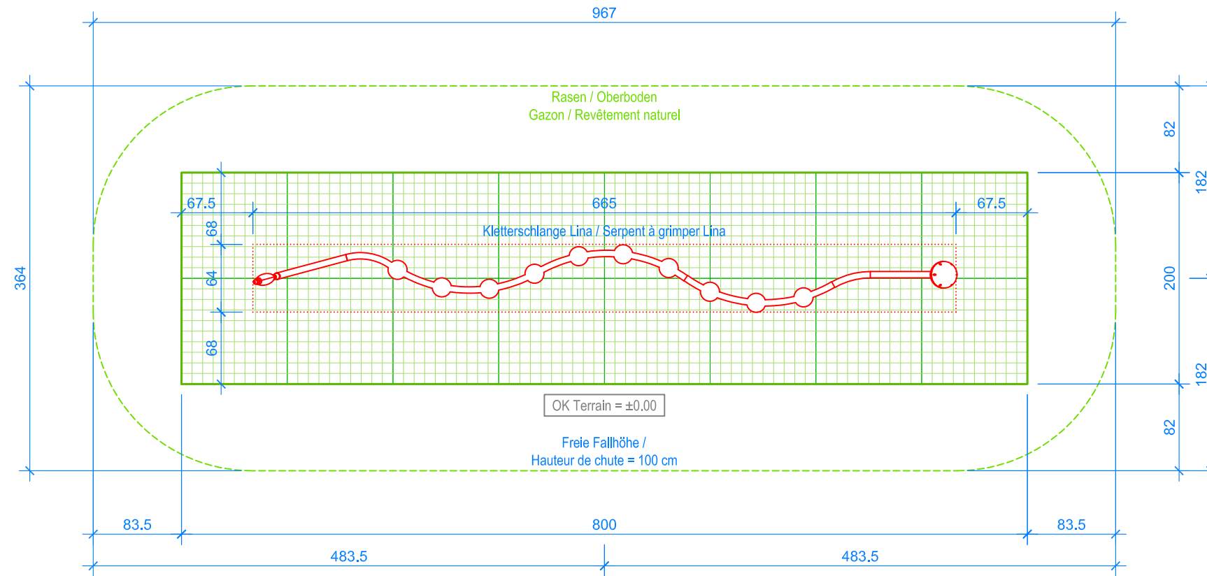
GRUNDRISS / PLAN 1:50
