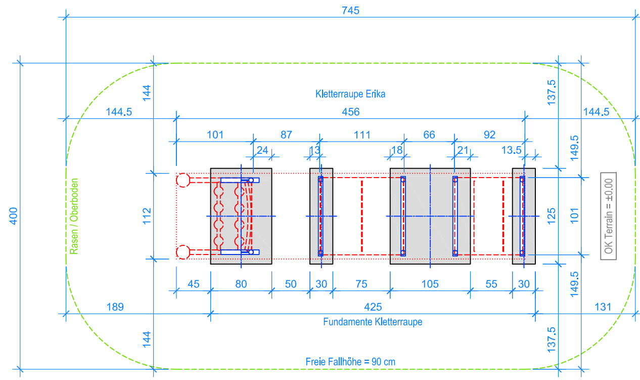
GRUNDRISS 1:50
