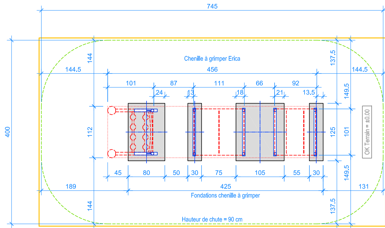
PLAN 1:50
