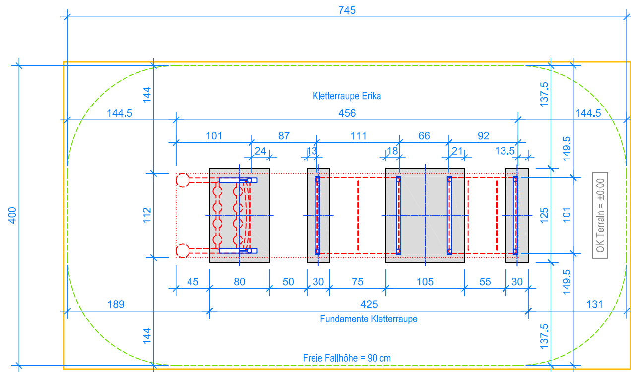
GRUNDRISS 1:50
