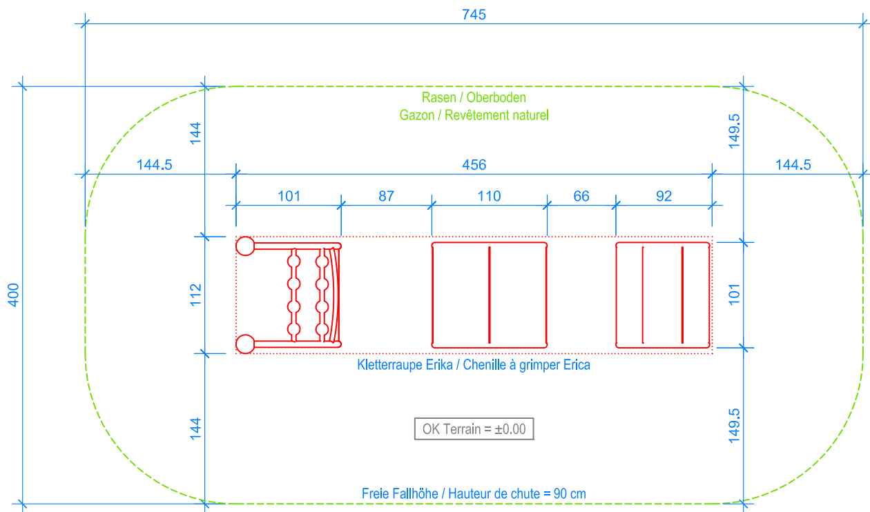
GRUNDRISS / PLAN 1:50
