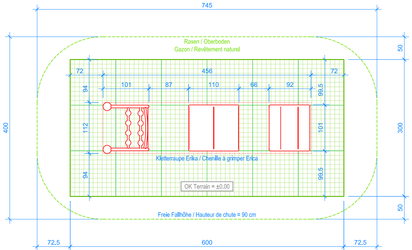
GRUNDRISS / PLAN 1:50
