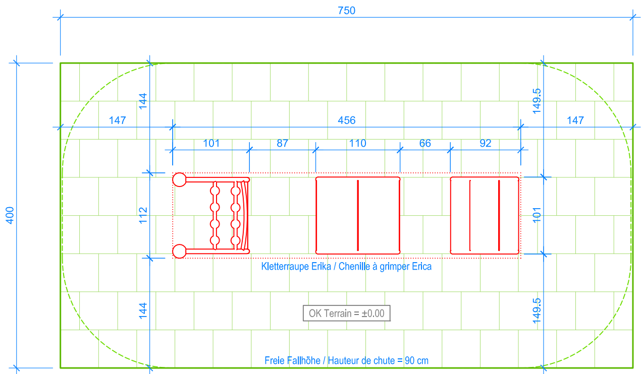
GRUNDRISS / PLAN 1:50
