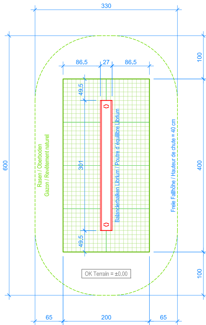
GRUNDRISS / PLAN 1:50
