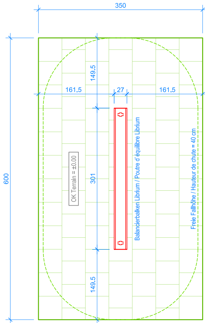
GRUNDRISS / PLAN 1:50
