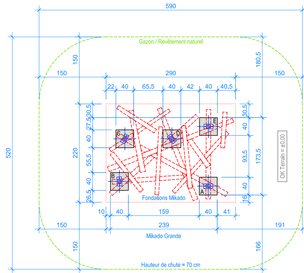
PLAN 1:50
