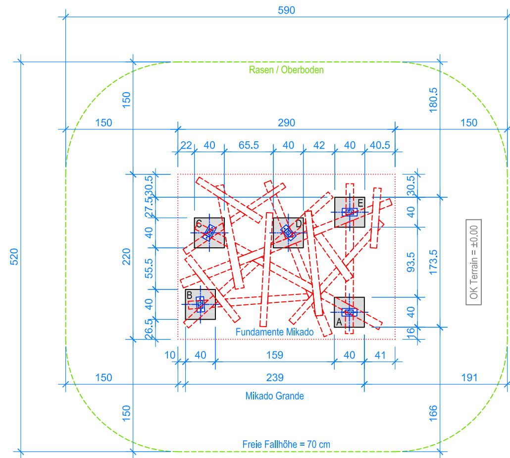
GRUNDRISS 1:50
