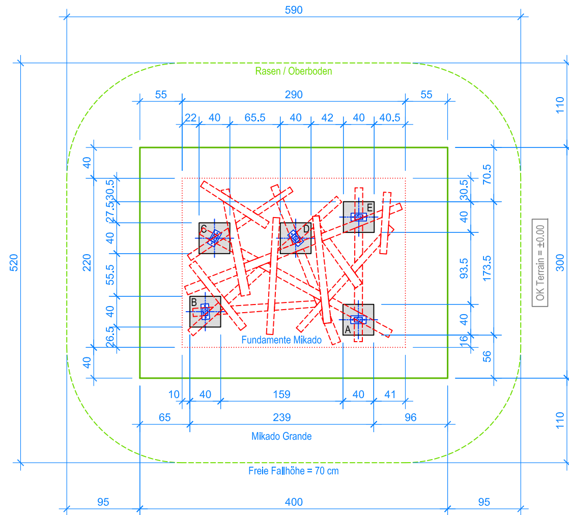
GRUNDRISS 1:50
