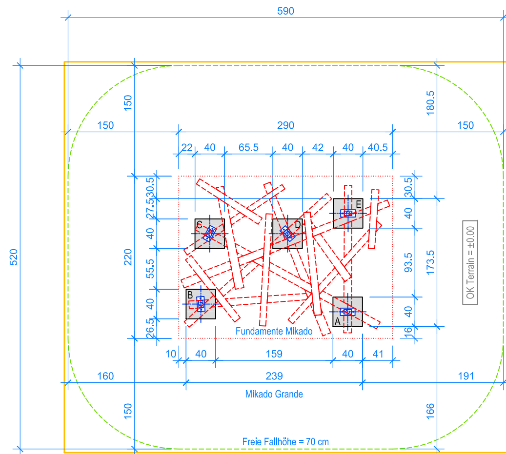
GRUNDRISS 1:50
