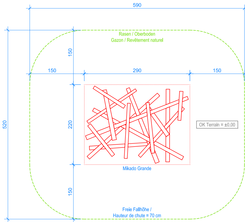
GRUNDRISS / PLAN 1:50
