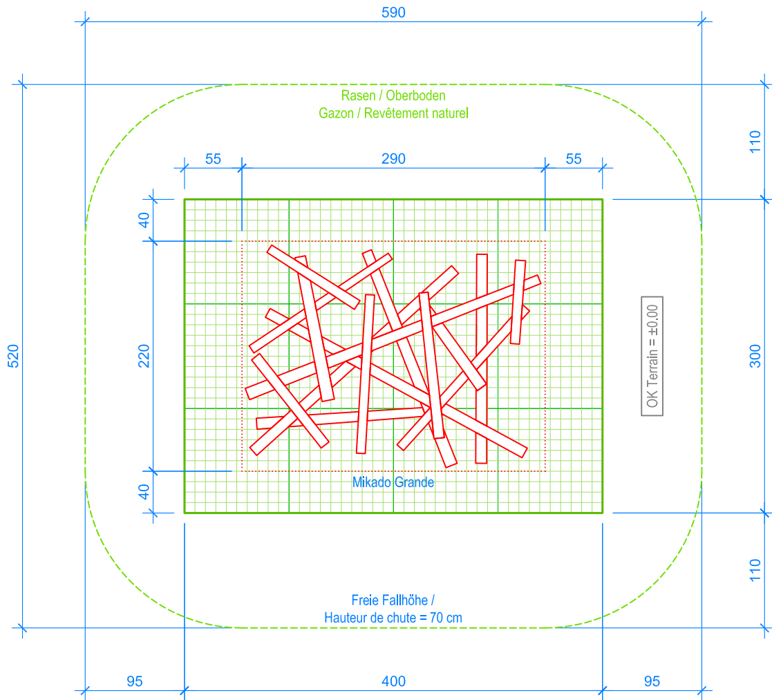
GRUNDRISS / PLAN 1:50
