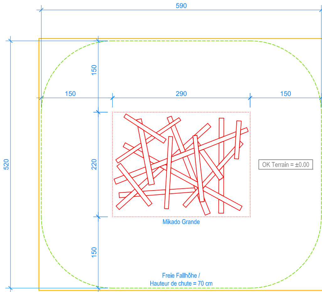
GRUNDRISS / PLAN 1:50
