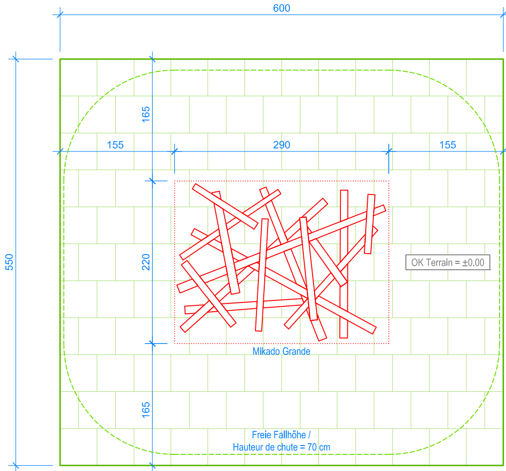
GRUNDRISS / PLAN 1:50
