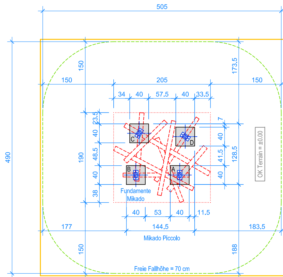
GRUNDRISS 1:50
