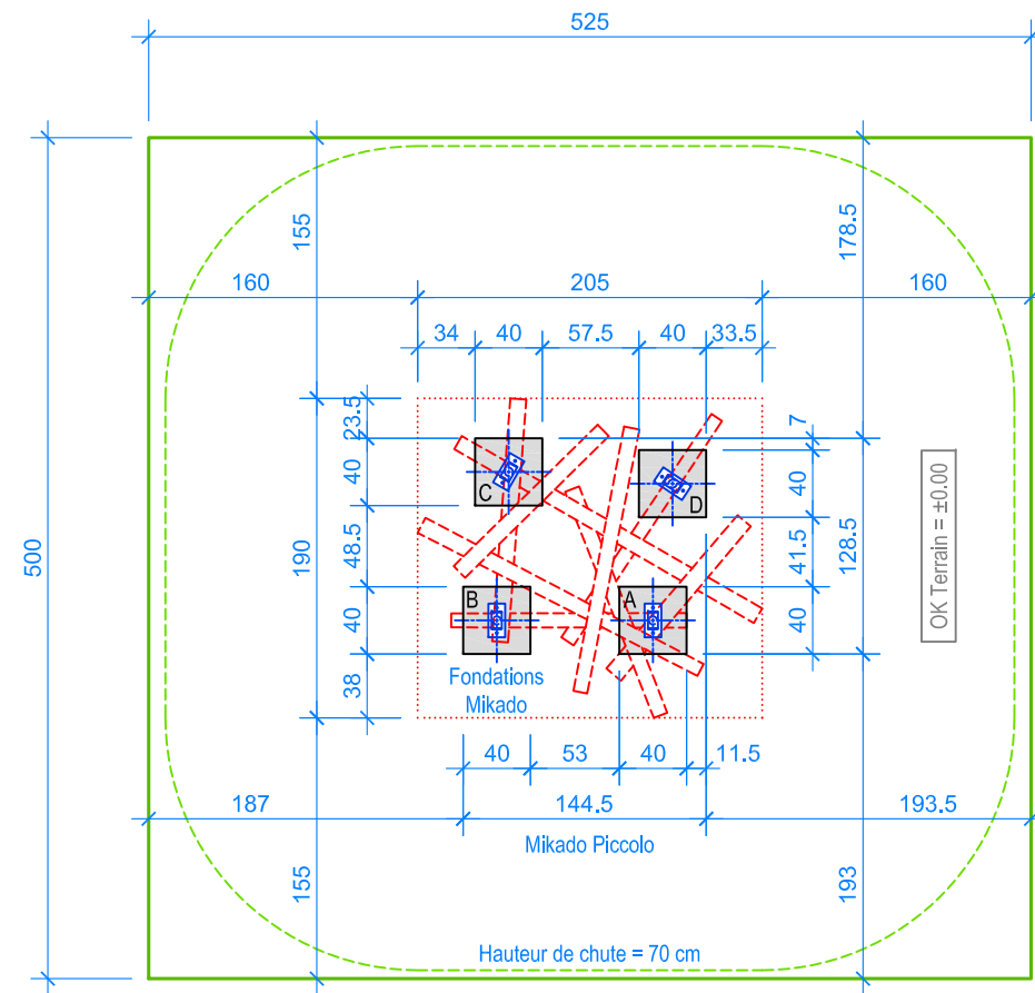
PLAN 1:50
