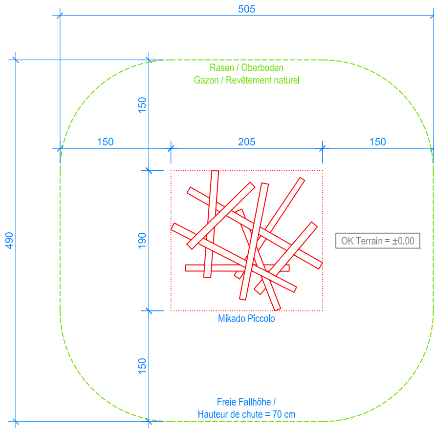
GRUNDRISS / PLAN 1:50
