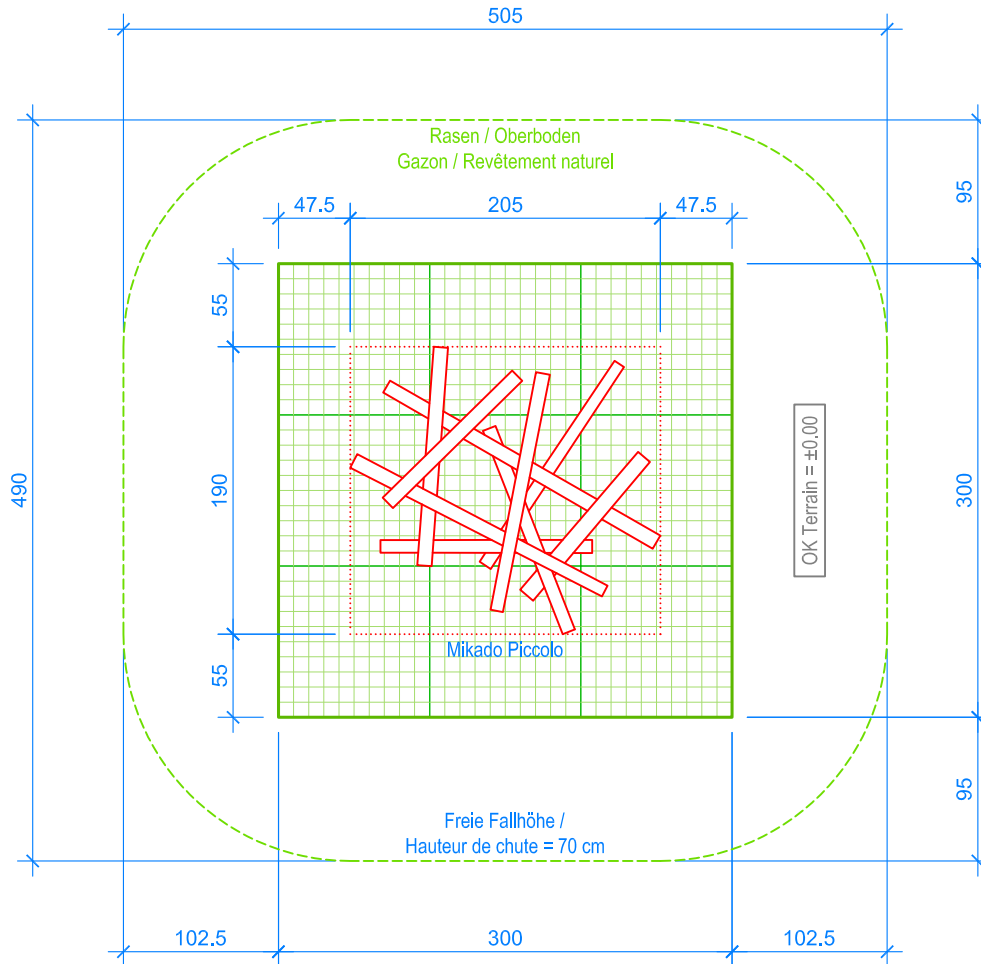
GRUNDRISS / PLAN 1:50
