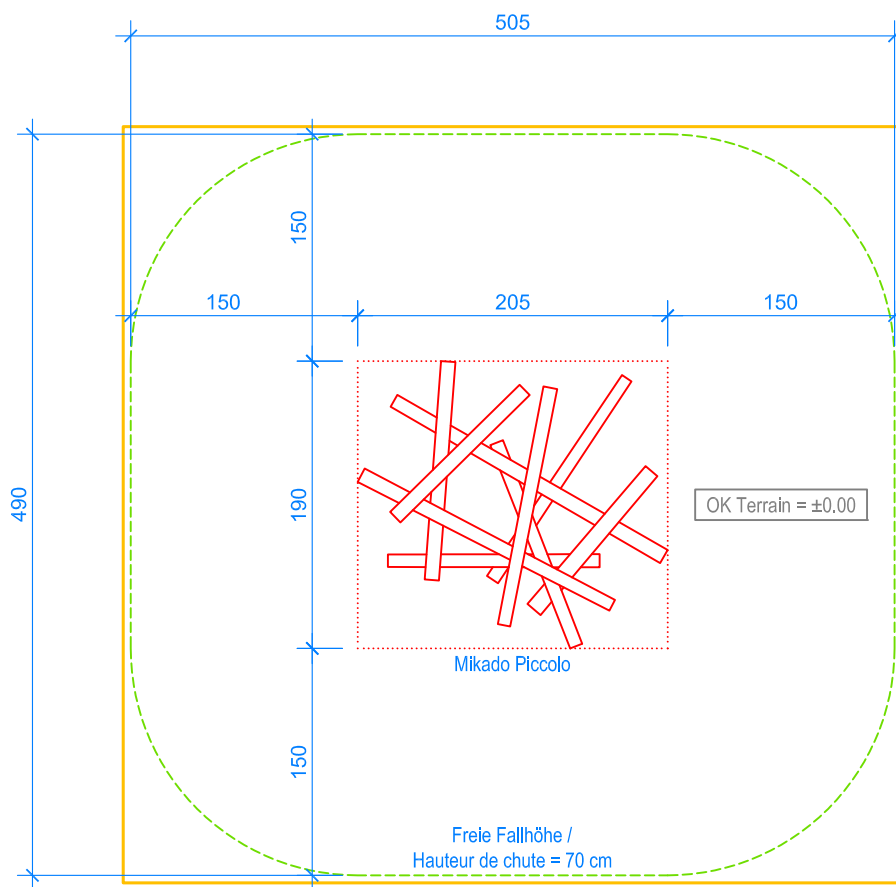
GRUNDRISS / PLAN 1:50
