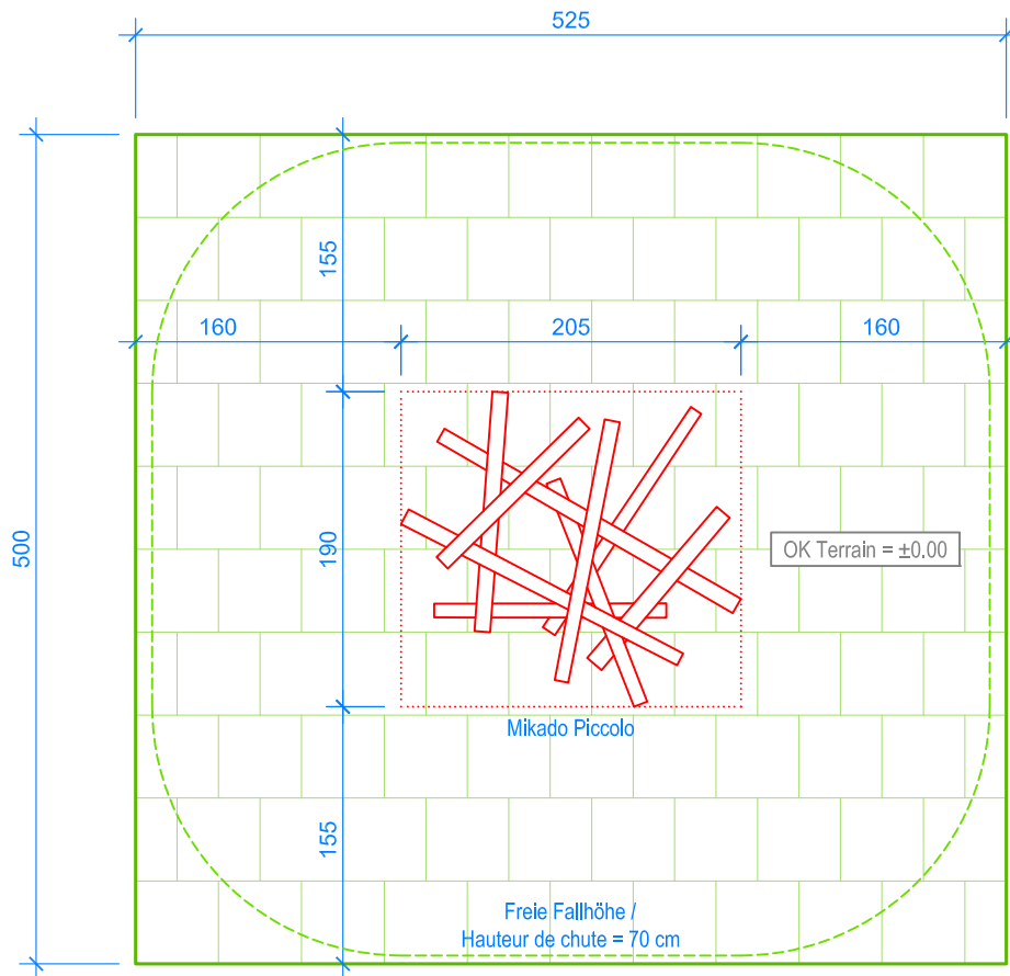
GRUNDRISS / PLAN 1:50
