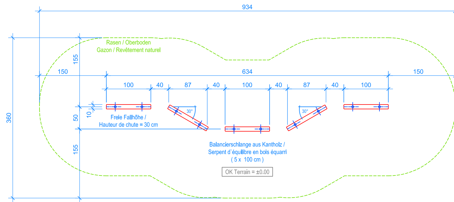
GRUNDRISS / PLAN 1:50
