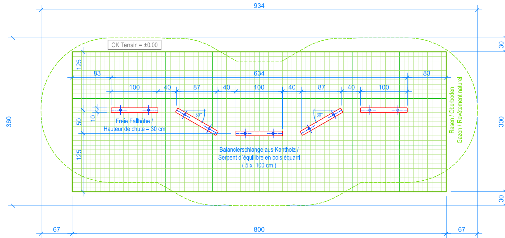
GRUNDRISS / PLAN 1:50
