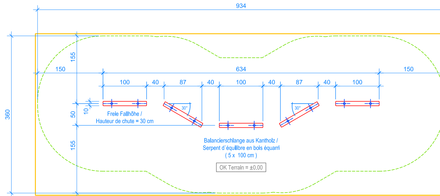
GRUNDRISS / PLAN 1:50
