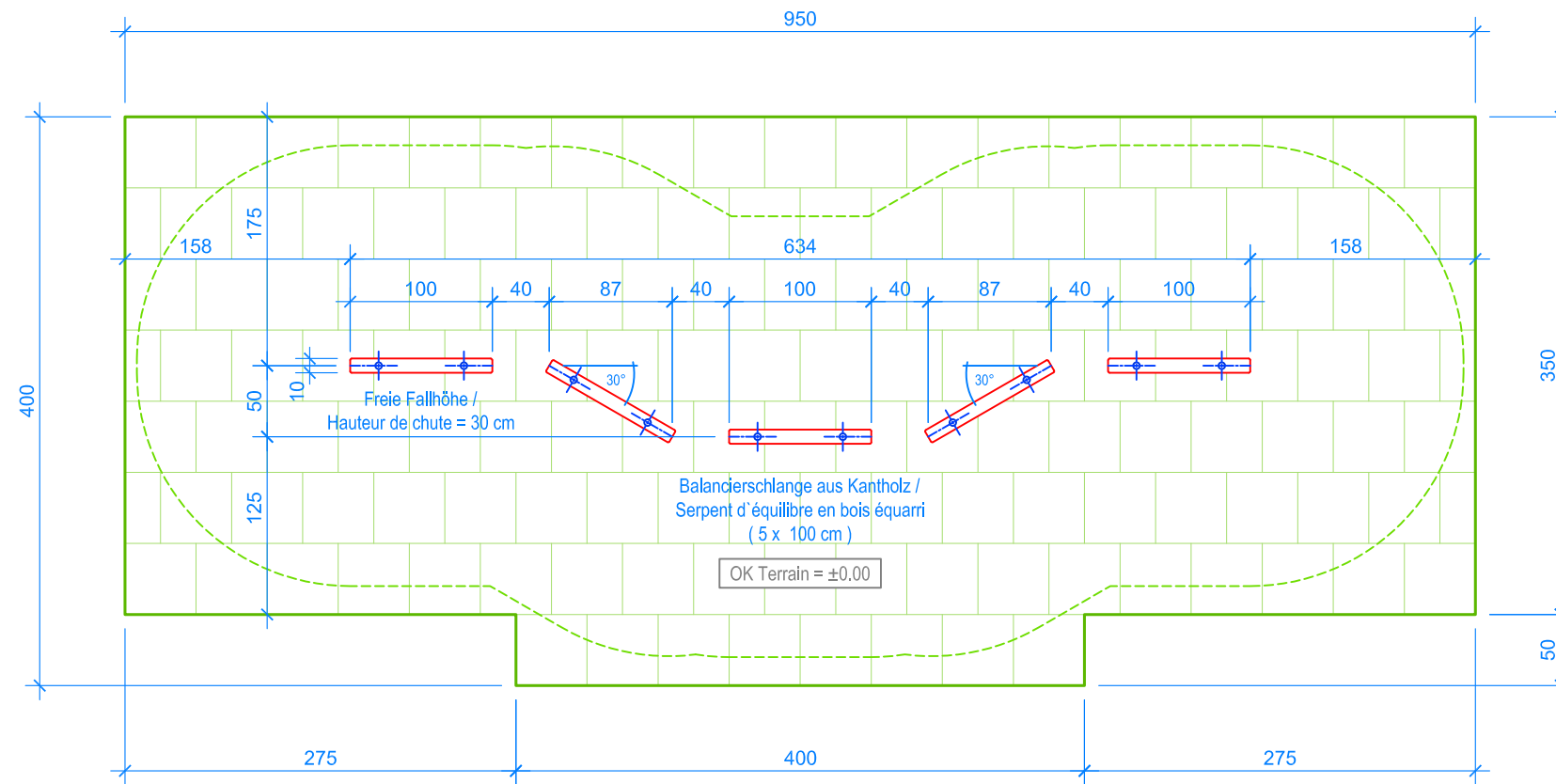
GRUNDRISS / PLAN 1:50
