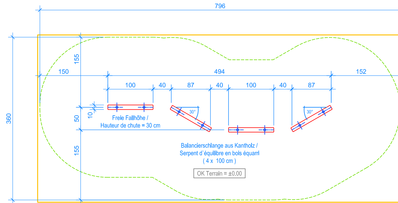
GRUNDRISS / PLAN 1:50
