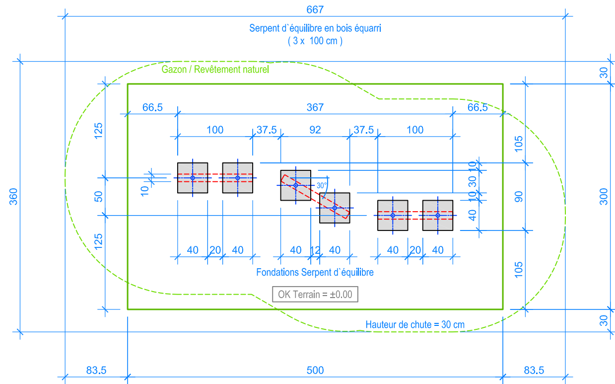
PLAN 1:50
