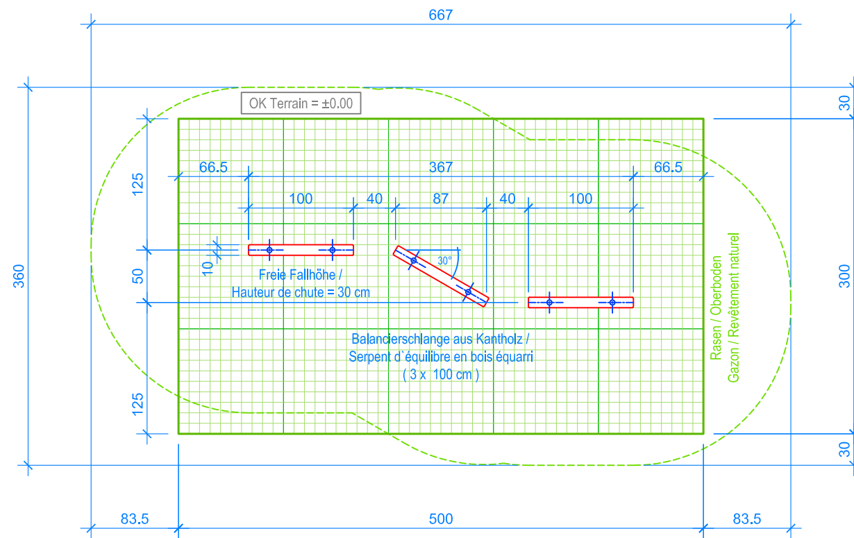
GRUNDRISS / PLAN 1:50
