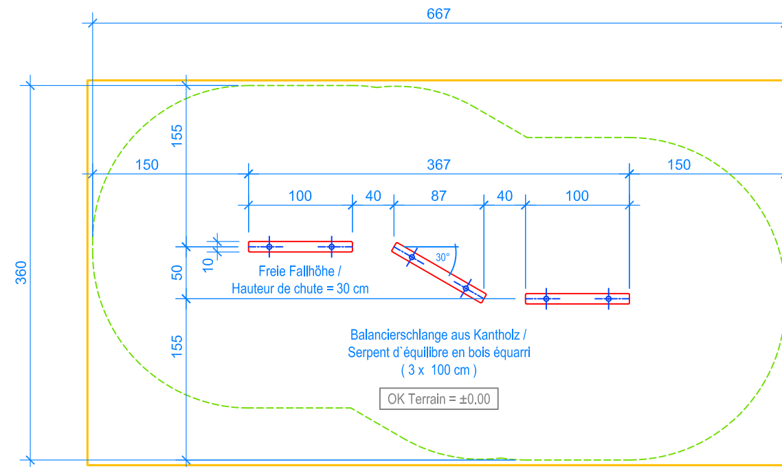
GRUNDRISS / PLAN 1:50
