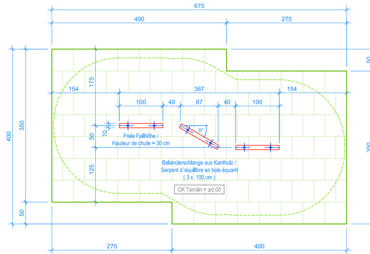
GRUNDRISS / PLAN 1:50
