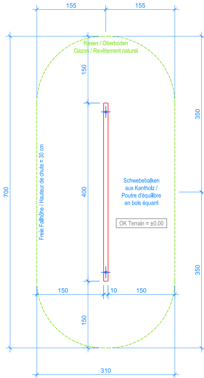
GRUNDRISS / PLAN 1:50
