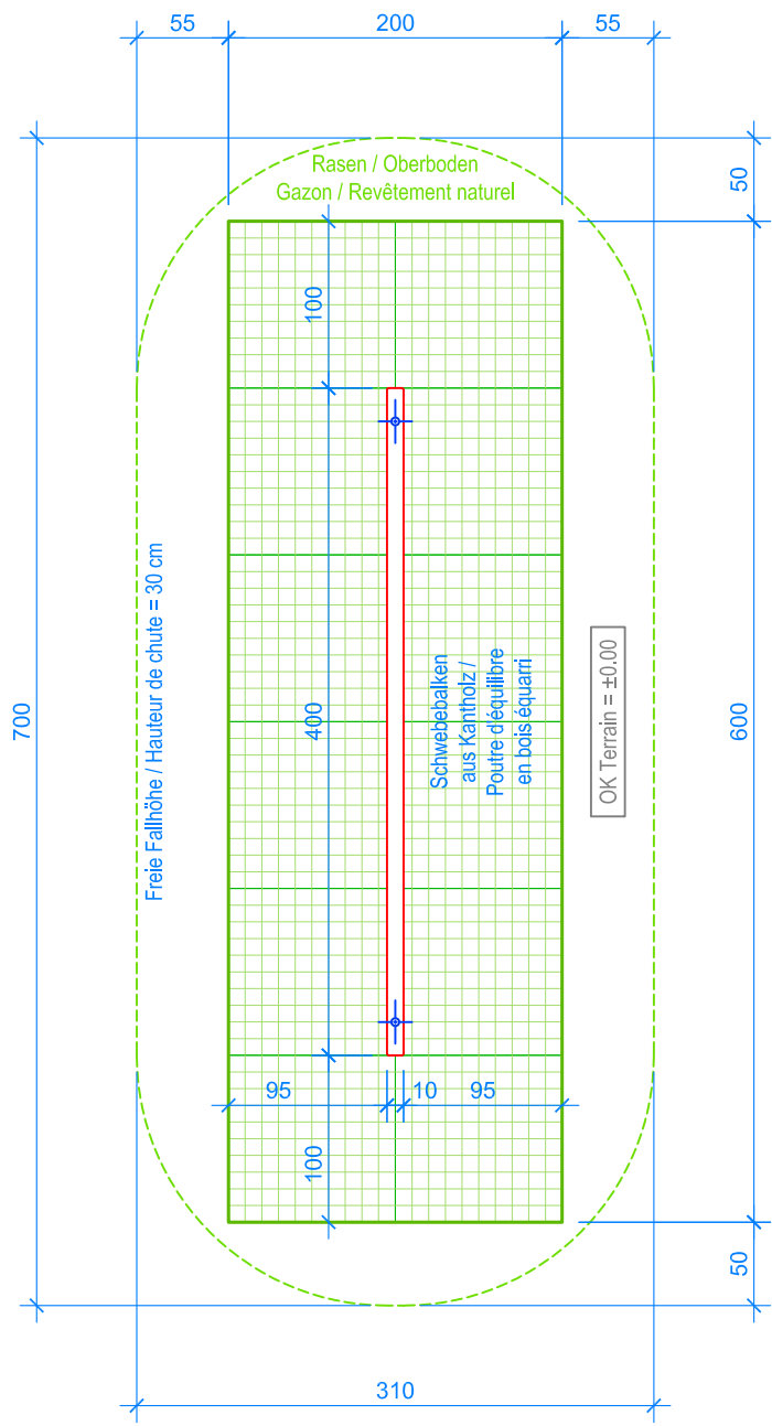
GRUNDRISS / PLAN 1:50
