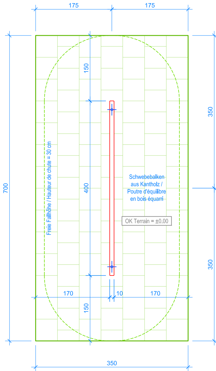
GRUNDRISS / PLAN 1:50
