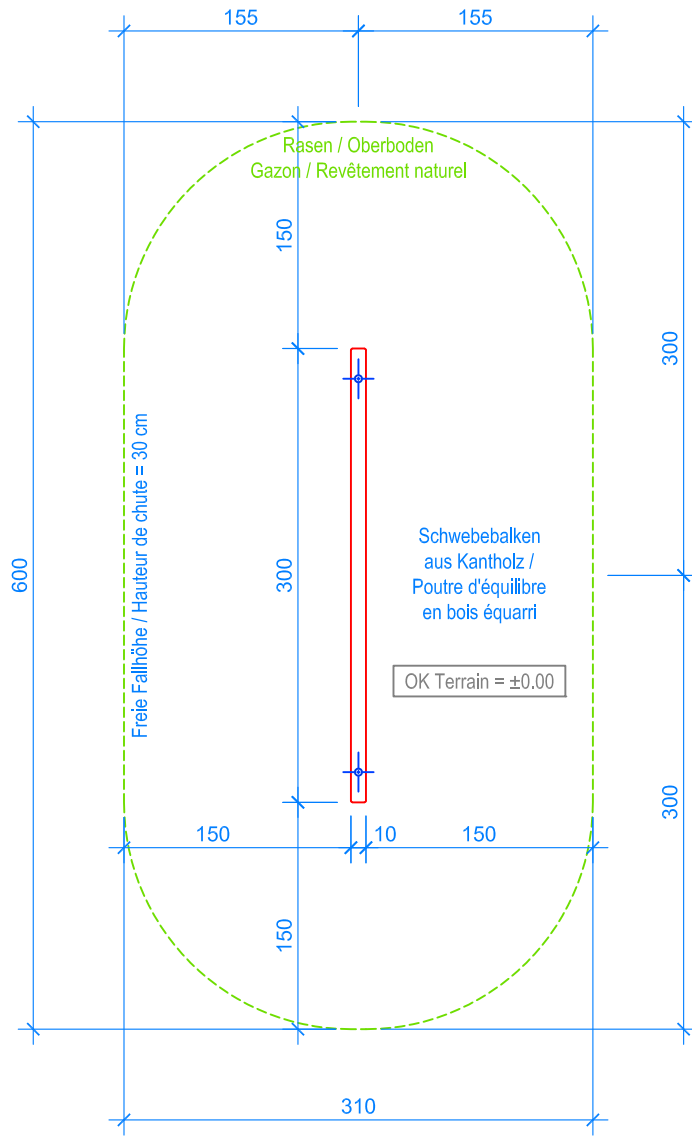
GRUNDRISS / PLAN 1:50
