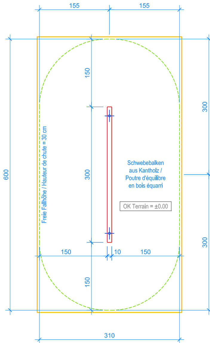
GRUNDRISS / PLAN 1:50
